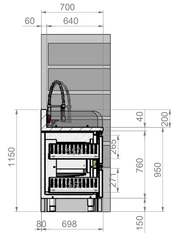
SEZIONE B-B
