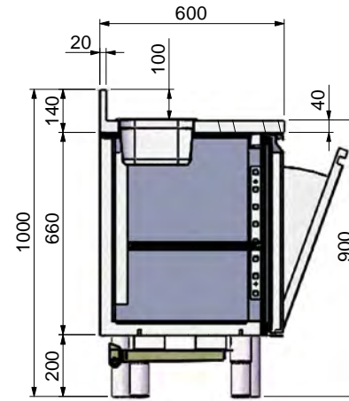
SEZIONE A-A
