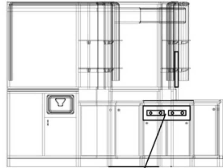
MEUBLE SUR MESURE POUR LOGEMENT MACHINES PLUS PROFOND DE 5 CM
