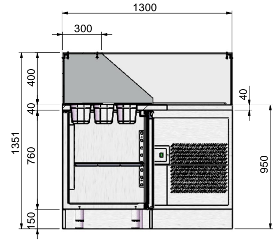
SEZIONE A-A
