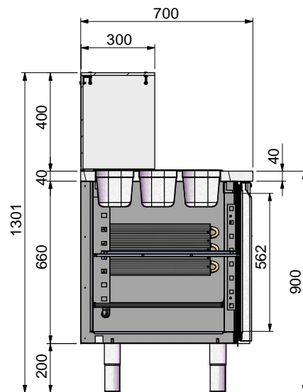
SEZIONE A-A
