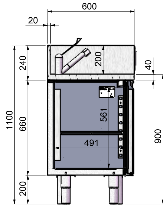
SEZIONE A-A
