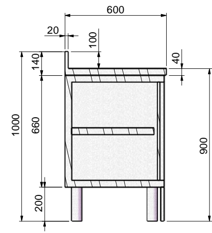
SEZIONE A-A
