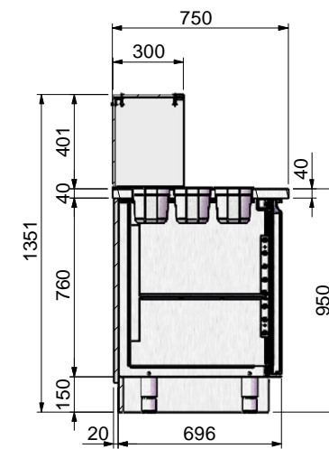
SEZIONE A-A
