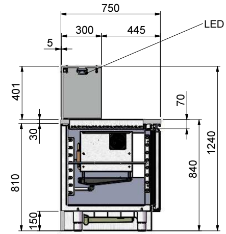
SEZIONE A-A
