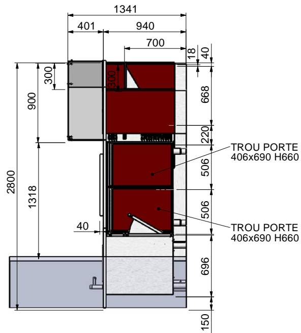
SEZIONE B-B
