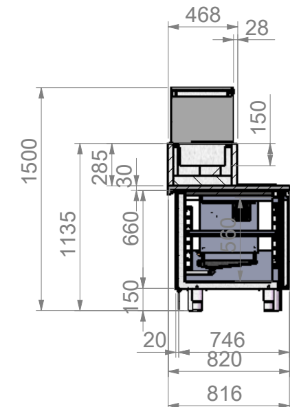
SEZIONE A-A
