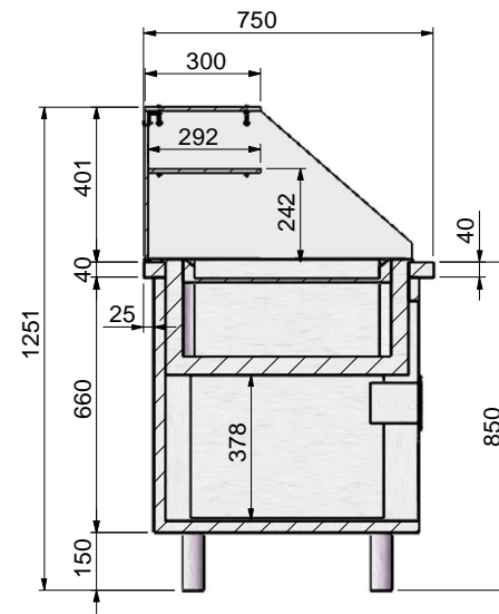
SEZIONE A-A
