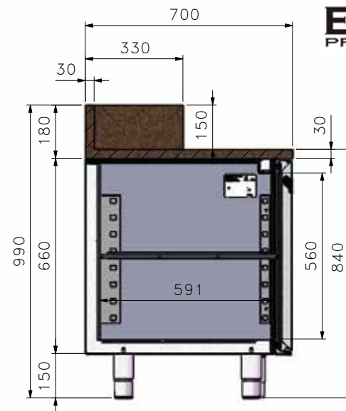
SEZIONE B-B
